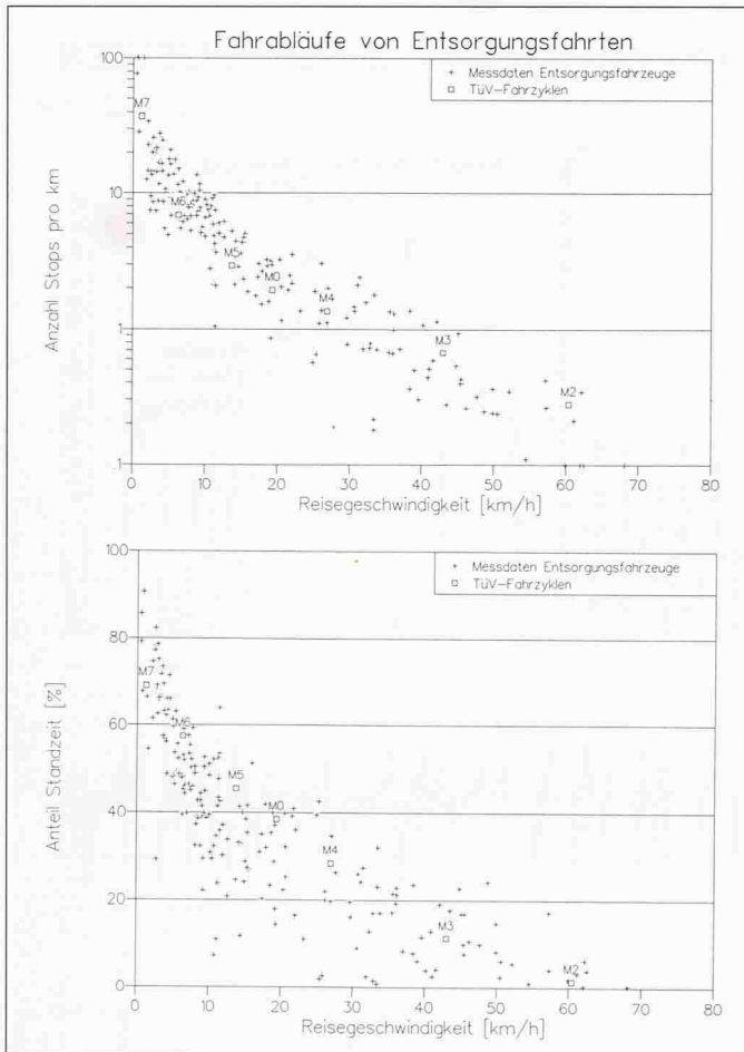
Bild 2. Vergleich der empirischen Fahrabläufe mit den TÜV-Fahrzyklen
