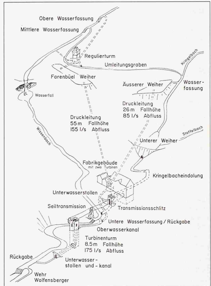
Bild 10. Schematische Perspektive des Wasserkraftsystems Neuthal entsprechend dem Konzessionsgesuch aus dem Jahre 1878. Der Kern der drei eigenständigen, aber eng ineinander verflochtenen Anlagen bestand aus Seiltransmission und zwei Turbinen im Fabrikgebäude, gespeist mit Druckleitungen vom Äusseren Weier bzw. vom Farenbuelweier.
