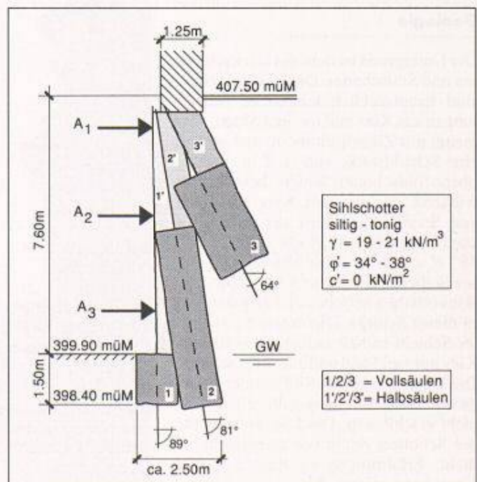
Bild 5. Schnitt A-A; Soilcetesäulen im Bereich Badenerstr. 4; Darstellung der Halb- und Vollsäulen
