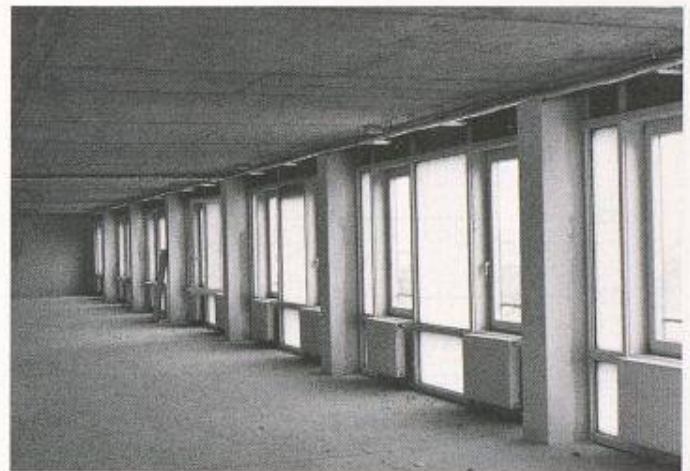
Bild 6. Transparente Isolation zur Tageslichtnutzung im Technologiepark Düsseldorf
