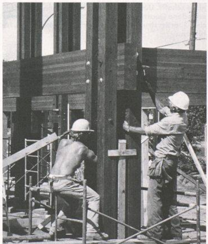
Bild 6. Mehrgeschossiges Bürogebäude mit Parallam-Stützen und Brettschicht-Unterzügen
