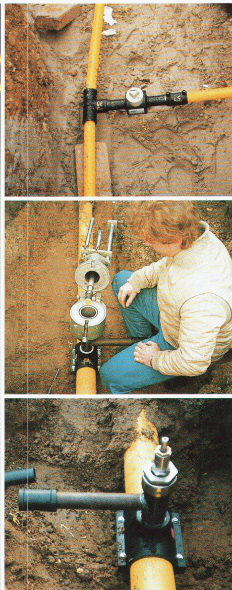
FRIALEN ® -Sicherheitsfittings liefern wir von d 20 – d 450
