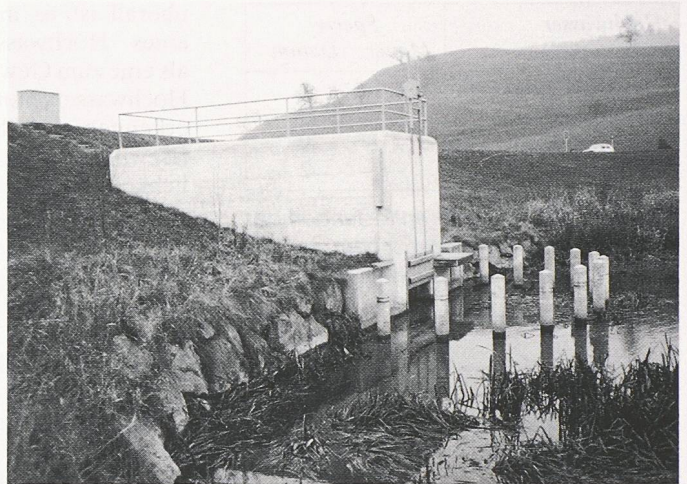
Bild 4. Hochwasserrückhaltebecken Turbenthal. Wasserseitige Dammböschung (Strassendam) mit Kombinationsbauwerk für Durchlass und Hochwasserentlastung; Betonpfähle als Grobrechen
