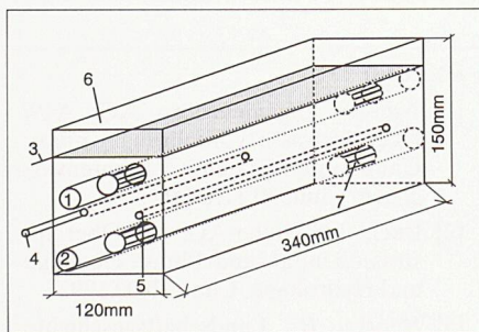
Bild 1. KKS-Prüfkörper aus Beton mit Anodennetz und Mörtelüberdeckung. – Beton: TFB-Standardbeton 0-16 mm, W/Z= 0.5, 300 kg PC/m 3 , 0.8% Sikament 300 (HBV), 0-4% Chlorid bezüglich Zement; – Mörtel: Labormörtel 0-5 mm (Normsand TFB), W/Z= 0.4, 450 kg PC/m 3 , 1.0% Sikament 300 oder Fertigmörtel mit und ohne Kunststoffzusatz; Legende: 1 – Stahlprobe Nr. 1, freie Länge: 300 mm, 2 – Stahlprobe Nr. 2, 3 – Anodennetz mit Anschluss, 4 – Bezugselektrode, 5 – Reserve-Öffnung für Bezugselektrode, 6 – Mörtel zum Einbetten der Anode, 7 – Kunststoff-Isolation, je 20 mm.
