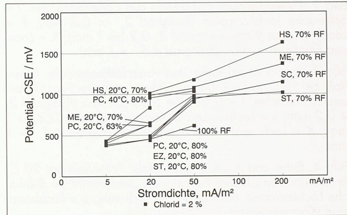
Bild 7. Anodenpotential: Ausschaltpotentiale in Funktion von Stromdichte, Klima
