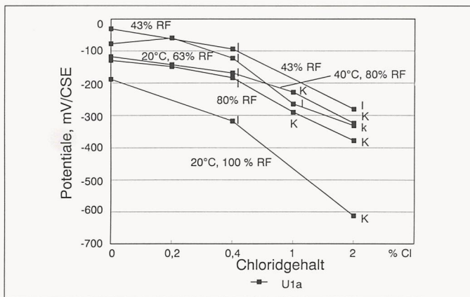
Bild 2. Ruhepotentiale in Funktion des Chloridgehaltes. l = Schwache Lochkorrosion (Rostgrad 2, < 0,2 mm); k = Lochkorrosion (Korrosionsgrad 3, 0,2 bis 1 mm); K = Loch- und Flächenkorrosion (Rostgrad 4,5, > 1 mm).
