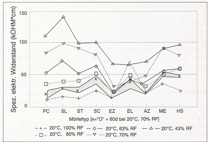
Bild 9. KKS-Mörtel, spezifische elektrische Widerstände nach 307 Tagen
