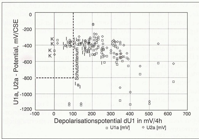
Bild 8. Depolarisationspotential dU_1 in Funktion der Ausschaltpotentiale U_{1a} , U_{2a} . l = Schwache Lochkorrosion (Rostgrad 2, < 0,2 mm); k = Lochkorrosion (Korrosionsgrad 3, 0,2 bis 1 mm); K = Loch- und Flächenkorrosion (Rostgrad 4,5, > 1 mm).
