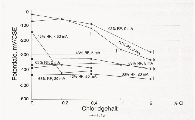
Bild 3. (rechts oben) Ruhe- und Ausschaltpotentiale. Potentiale bei 20 C, in Funktion von Chlorid, relativer Feuchtigkeit und Stromdichte. l = Schwache Lochkorrosion (Rostgrad 2, < 0,2 mm); k = Lochkorrosion (Korrosionsgrad 3, 0,2 bis 1 mm); K = Loch- und Flächenkorrosion (Rostgrad 4,5, > 1 mm).
