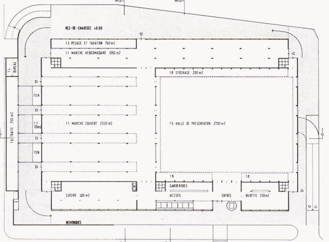
rez-de-chaussée
