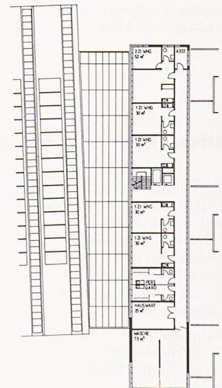
Erdgeschoss 2. Obergeschoss
