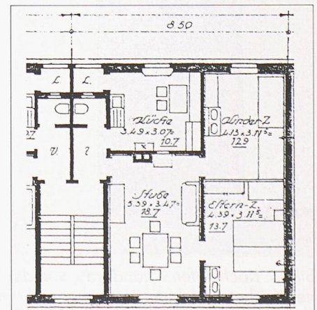
Bild 3. Grundriss einer typischen 4-Zimmer-Wohnung
