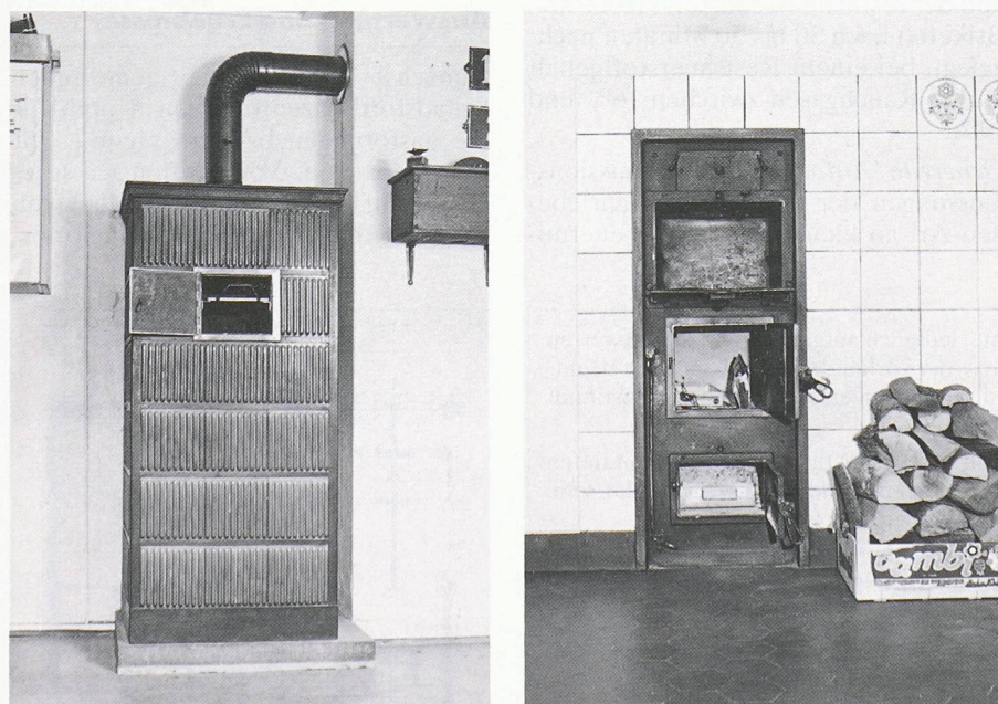
Bild 4. Kachelofen «Standard», von der Stubenseite her betrachtet: einfacher grüner Kachelmantel und Warmhalterohr mit Messingtüre (links); Kachelofen «Standard», Kücheenseite: schwarze Metallfront mit Kochrohr (oben), Feuerraum mit Metallrost (Mitte) und Aschenschublade (unten). Zuluftregulierung über die «Rosetten» in den beiden unteren Türen (rechts).
