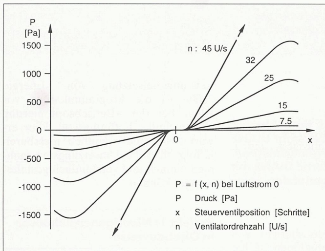
Bild 2. Steuerventilcharakteristiken (SVC)
