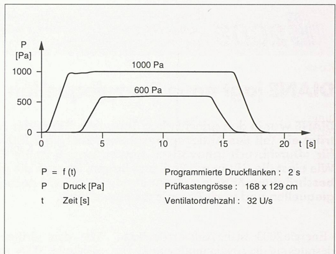
Bild 3. Druckpulse
