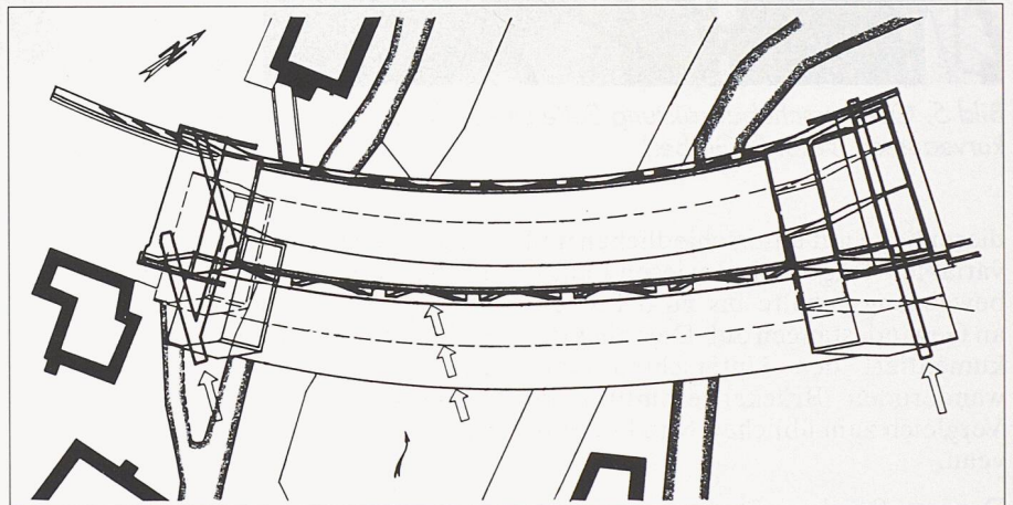
Bild 1. Disposition des Querverschubes der Landquartbrücke (Ing.büro H. Rigidinger)
