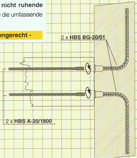
Grundriss-Detail
