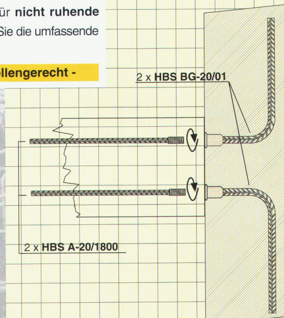
Grundriss-Detail
