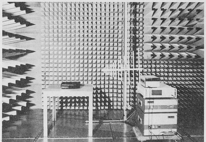
Bestehender Absorberraum der EMC Fribourg
