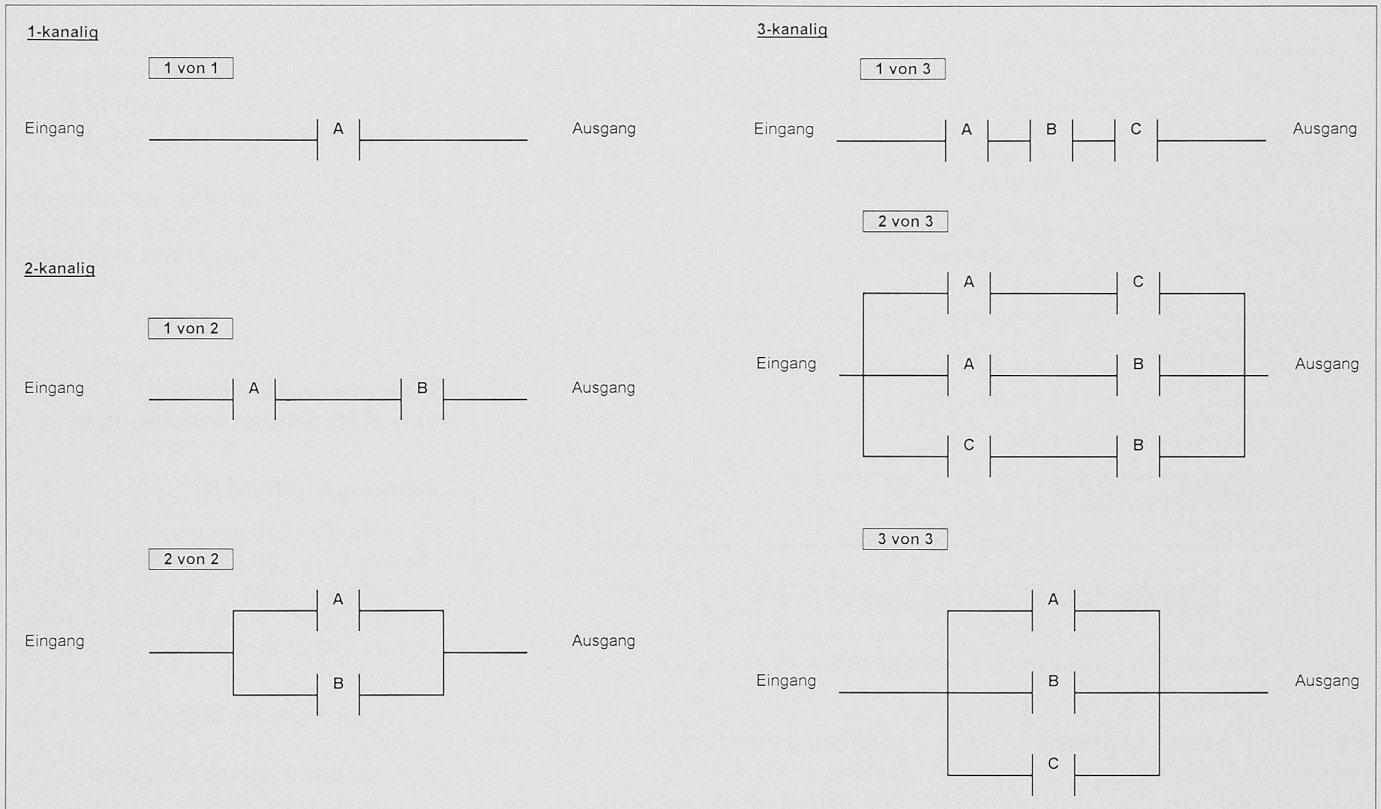
Bild 6. Grundschaltungen mittels m-von-n-Bewertung
