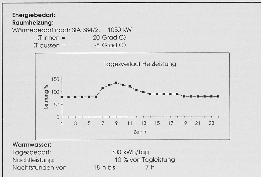
Bild 1. Eingaben Energiebedarf
