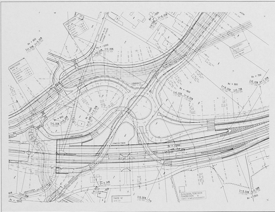
Bild 3. Der neue Autobahnanschluss Luzern-Horw wird erstmals in der Schweiz als Kreisbauwerk ausgebildet. Neben den vier Anschlussspuren laufen auch die drei Zubringerstrassen beim Kreisel «Schlund» zusammen. Der abgebildete Plan wurde, wie das gesamte Erweiterungsprojekt, mit dem CAD-Programm STRATIS konstruiert und gestaltet
