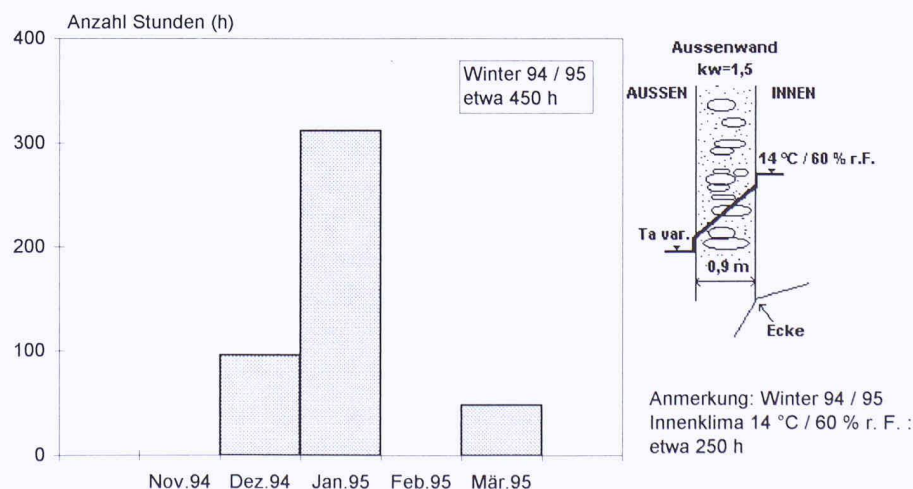
Bild 2. Unterschreitung der Taupunkttemperatur (h) an Aussenwanddecke. Innenklima: 14 °C/60% r.F. Aussenklima: Stadt St.Gallen. Ablesebeispiel: Während des Monats Januar 1995 kam es an
