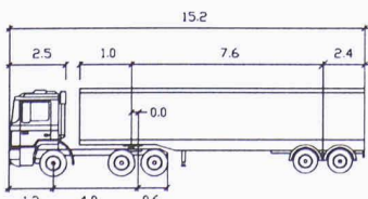
SATTELSCHLEPPER
