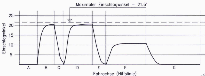
Bild 1. Betonung des Eckverkehrs B-C, Dämpfung der Fahrgeschwindigkeit A-C mit minimalem Flächenbedarf. Bewegungsfälle für Fahrbeziehungen: A-B und A-C Lastwagen Typ B, B-C Lastwagen mit Anhänger Typ B in allen Fällen für beide Fahrrichtungen gemäss [2]
