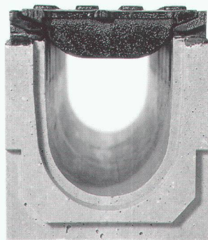
Eine ACO-Innovation: kompakter auf extremste Belastungen ausgelegter Rinnenkörper mit schraubenloser Arretierung.
