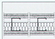
Hohe Dämmung: FERMACELL Montagewand 1 S 31, Stahl-Unterkonstruktion, doppelt beplankt. R_{w,R} 57 dB, F 90-A.
