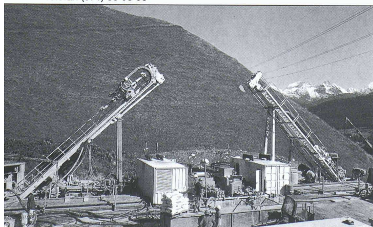
baustelleneinrichtung für die Foralith-Tiefbohrungen.
