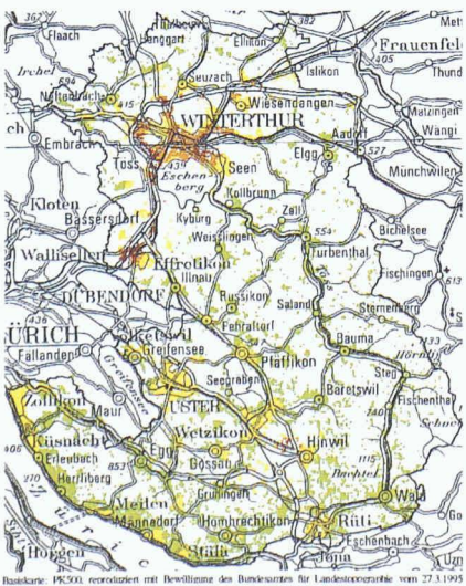
Schadstoffkonzentrationen und -depositionen in der Raumplanung Von NO 2 - Konzentrationen betroffene Einwohner unter dem Grenzwert in der Höhe des Grenzwertes bis unter 50 % über dem Grenzwert 50 % oder mehr über dem Grenzwert
