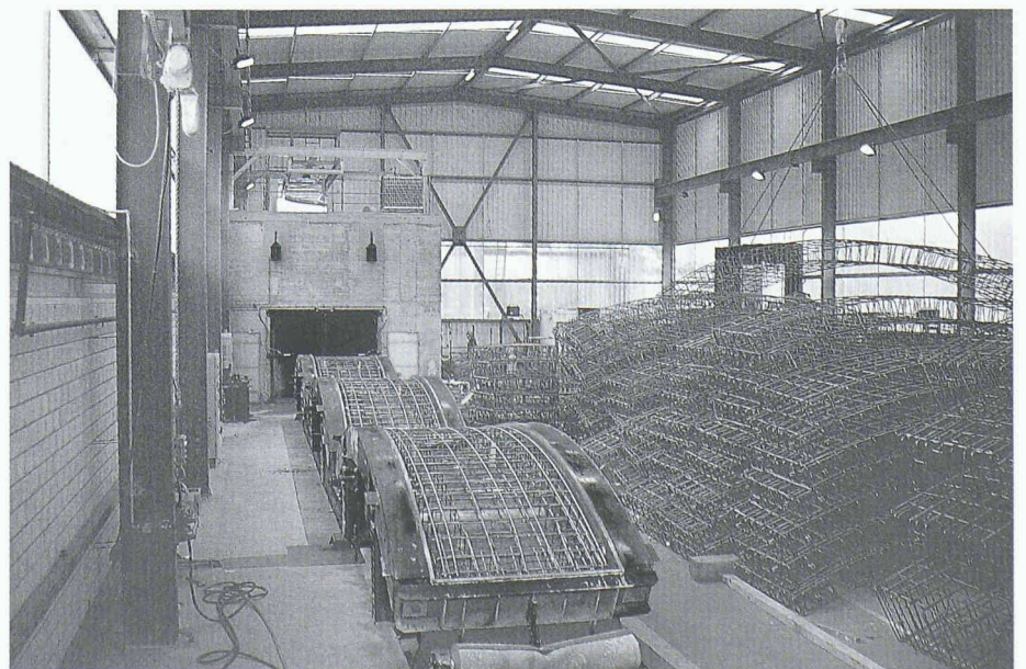
Tübbingfabrikation
