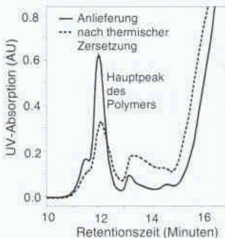
5 Chromatogramm eines Polymerbitumens vor und nach thermischer Zersetzung
