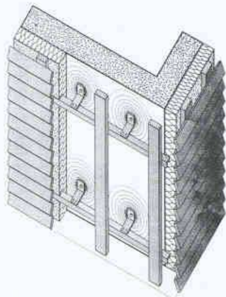
2 Unterkonstruktion in Stahl oder Aluminium mit Konsolen und Winkelprofil zur Befestigung des Wetterschildes (Bild: Hans Bertschinger, Empa-KWH)
