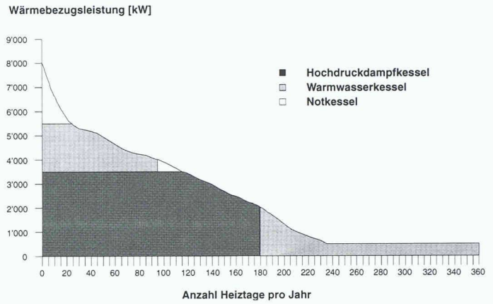
Lastdiagramm des Heizkraftwerkes Meiringen. Der Hochdruckdampfkessel ist im Winterhalbjahr, der Warmwasserkessel im Sommerhalbjahr sowie während 90 kalten Tagen in Betrieb [4]
