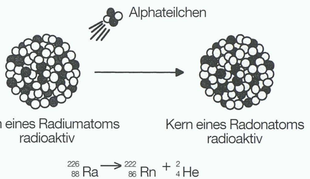
6 Umwandlung von Radium zu Radon
