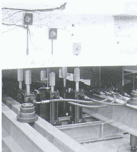
Verteilte Lasteinleitung beim Versuchsträger EB4
