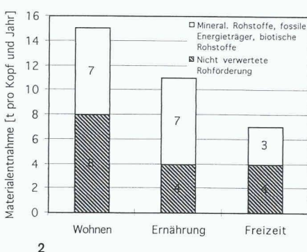
2 Materialentnahme nach Bedarfsweldern (Quelle: Behrensmeier und Bringezu, Wuppertal Institut für Klima, Umwelt, Energie, 1995, Graphik: R. Coutalides)
