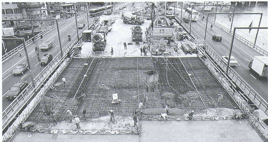
4 Dritte Betonieretappe
