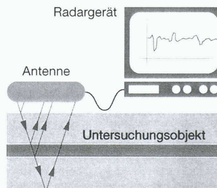
Funktionsprinzip des Georadar
