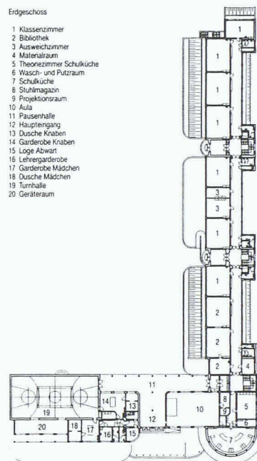
Erdgeschoss
