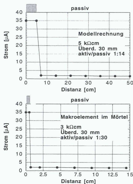
Stromausbreitung bei lokaler Korrosion: Vergleich der Resultate am Modell-Makroelement mit Simulationsrechnungen
