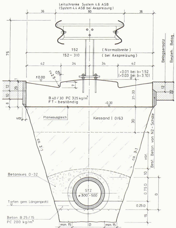
1 Normalquerschnitt der neuen Hauptleitung im Mittelstreifen
