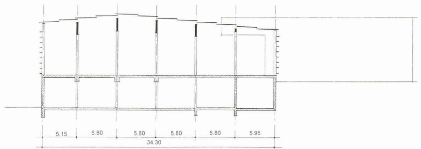
2 Längsschnitt
