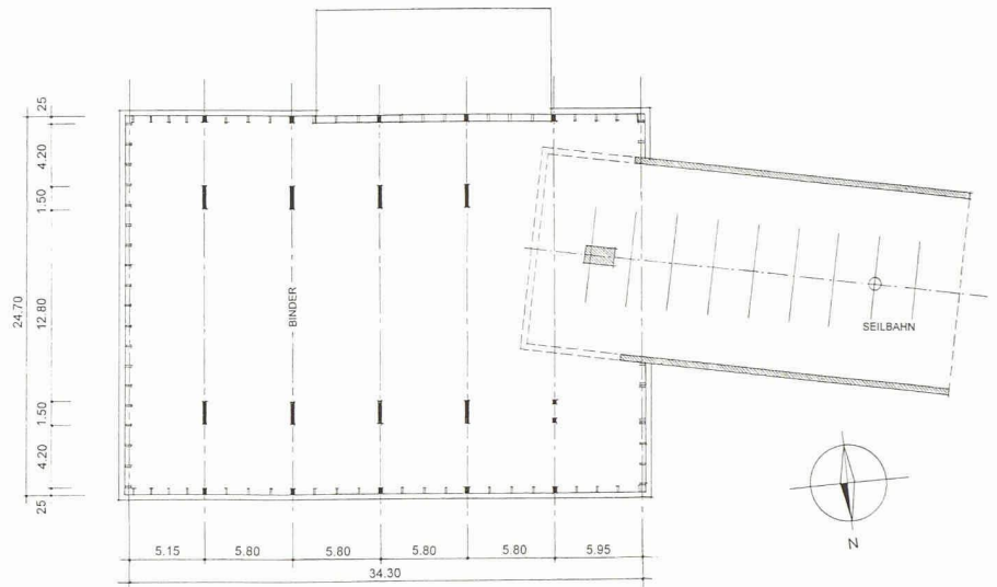
1 Grundriss Halle
