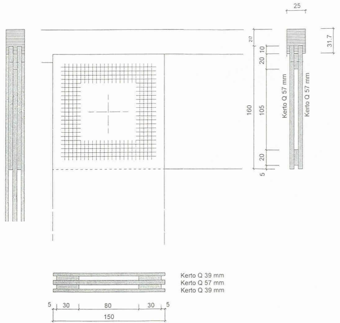
4 Detail eines Rahmenecks
