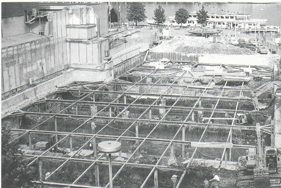
Ausgesprissste Baugrube (Bild: J. Brun, Luzern)
