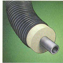
Biegerohrsystem, Flexopan-Stahl
