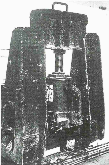
Selbst entwickelte Vorspannpress mit einem Lastwagenheber als Kernstück
