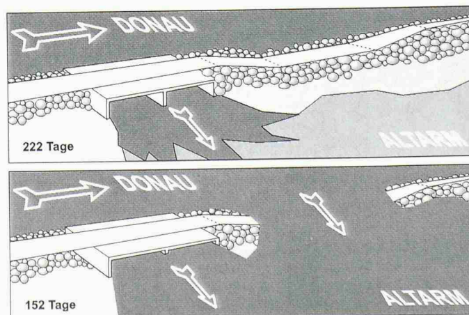
1 Die Kombination von Durchlässen und Überstrombereichen sorgt für dynamische Fließverhältnisse in den Auengewässern
