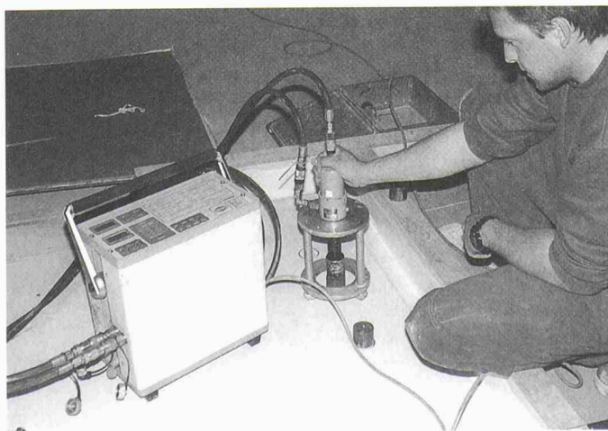
Der Verband Schweizer Industrieboden-Unternehmer (VSIU) hat eine Qualitätsprüfung für Industrieböden erarbeitet. Eines der Kriterien ist die Haftzugfestigkeit, die hier getestet wird
