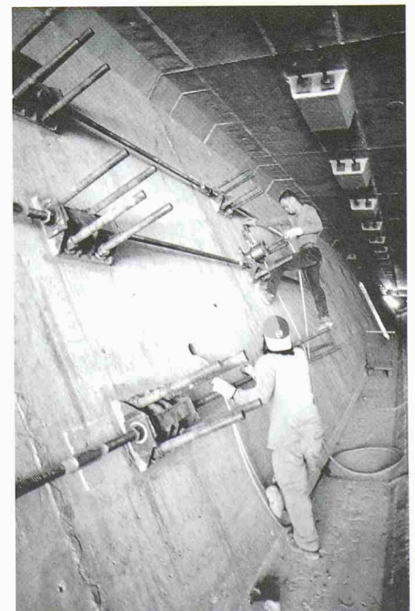
11 Typische Anordnung der temporären Vorspan- nung
