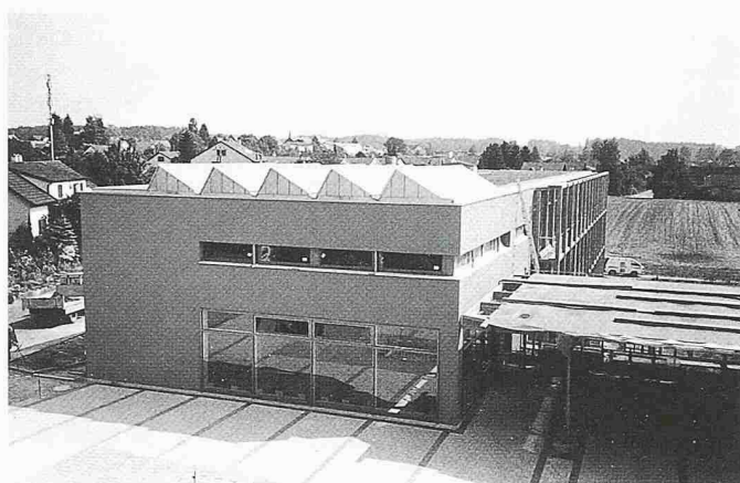
Erweiterungsbau des Oberstufenzentrums Berg TG mit Blech-Sheddach (Vordergrund) und extensiv begrüntem Foamglas-Gefälledach
