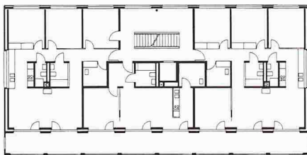
3 Grundriss Obergeschoss
