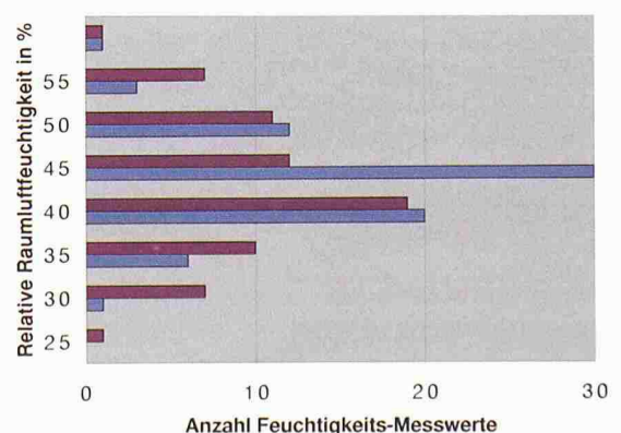
Häufigkeitsverteilung der Luftfeuchtigkeits-Messwerte während der Heizperiode (monatliche Momentanwerte aller Wohnungen). Legende: blau 97/98; rot 98/99
