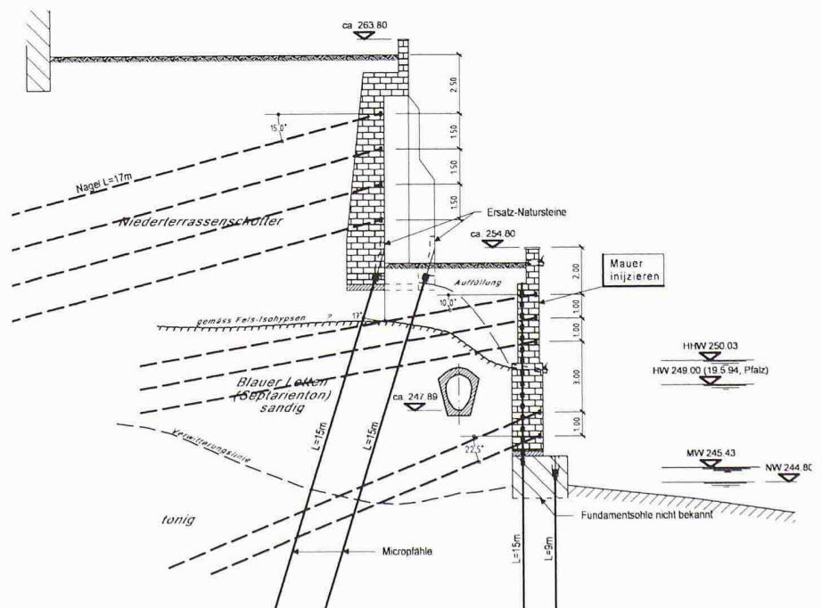
6 Abschnitt Hohenfirstenhof, Vernagelung und Micropfähling
