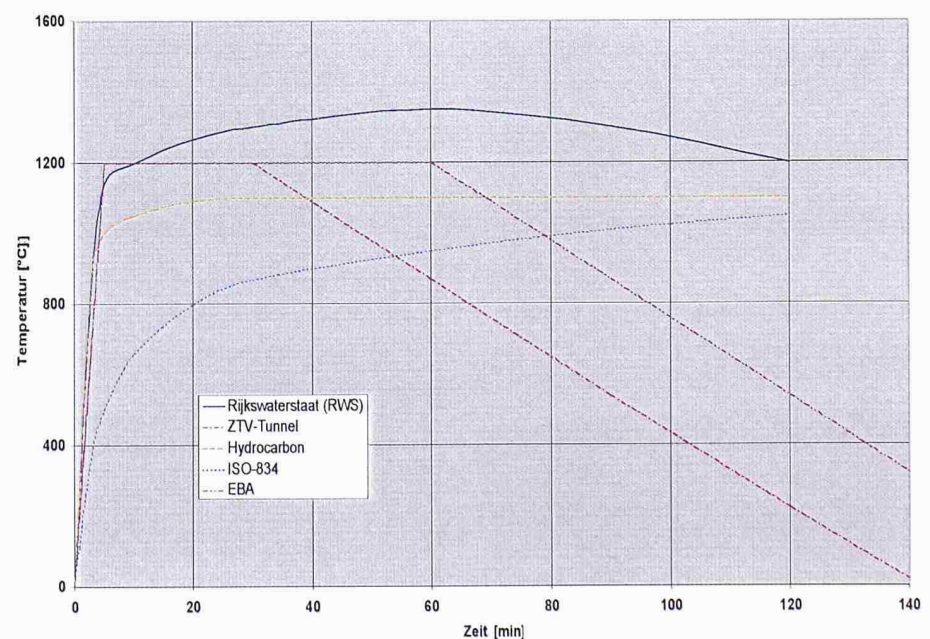
3 Brandlastverläufe
