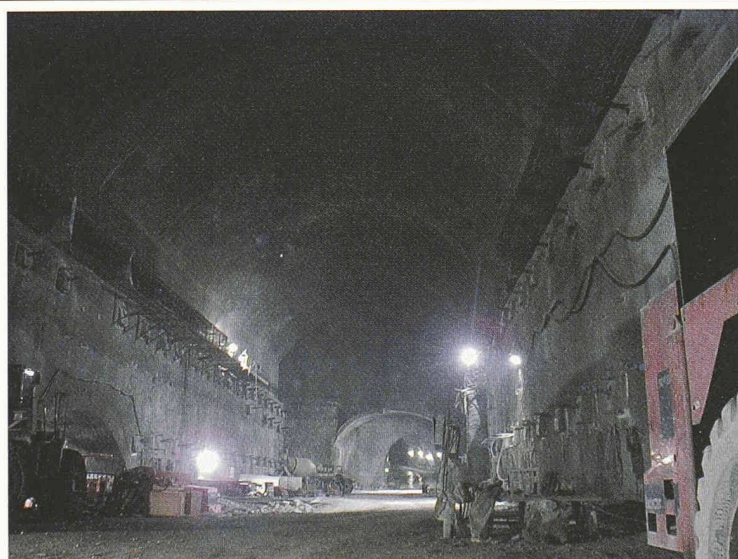
Aufnahme bei Halbzeit der Ausbruchsarbeiten der Zentrale Deriner – Türkei ( H = 25 m, B = 30 m, L = 120 m )
