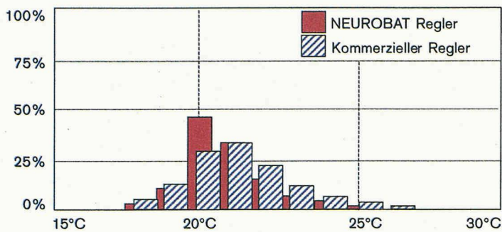
Komfortquantifizierung im Vergleich: Die gemessenen Raumtemperaturen während der Benutzerpräsenz, Sollwert 20 °C
